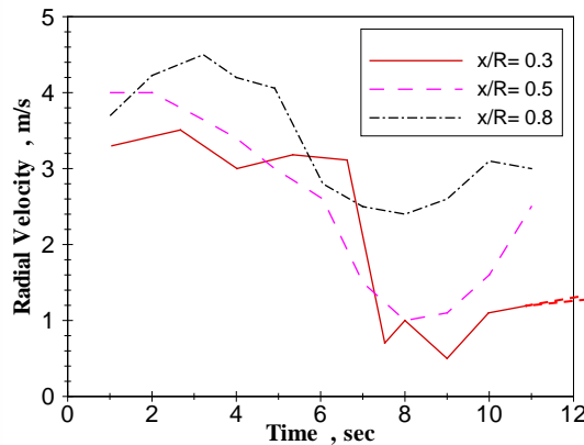
شکل ۱ - تغییرات سرعت شعاعی نسبت به زمان (فونت: BZar 9 pt, Bold) (اندازه فونت ۹ و ضخیم)
